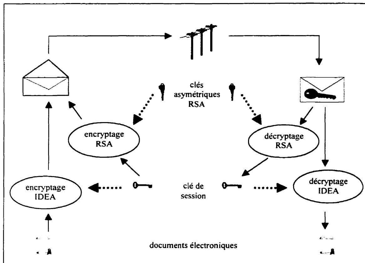
Figure 4.14 – Le transport et la protection des enveloppes virtuelles
